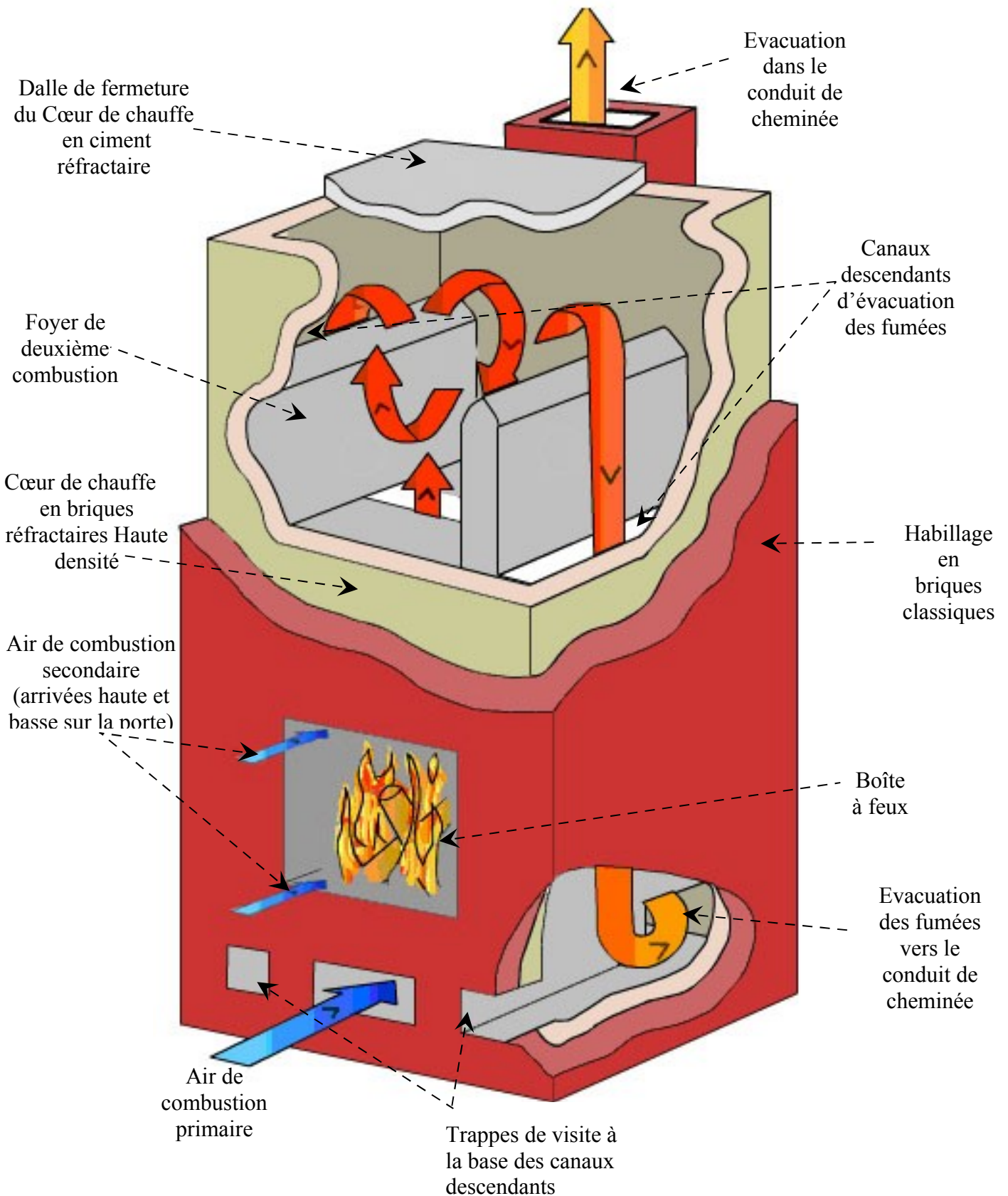
Schéma de fonctionnement d'un foyer de masse de style finlandais.
